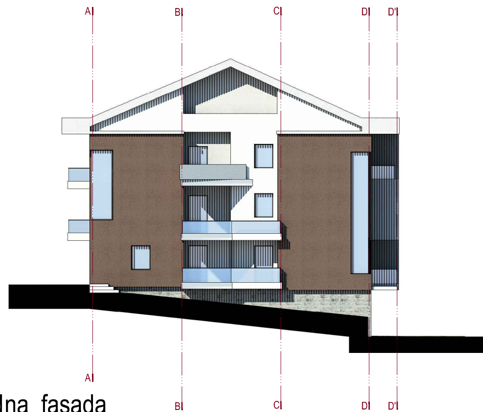
jugoistočna fasada
